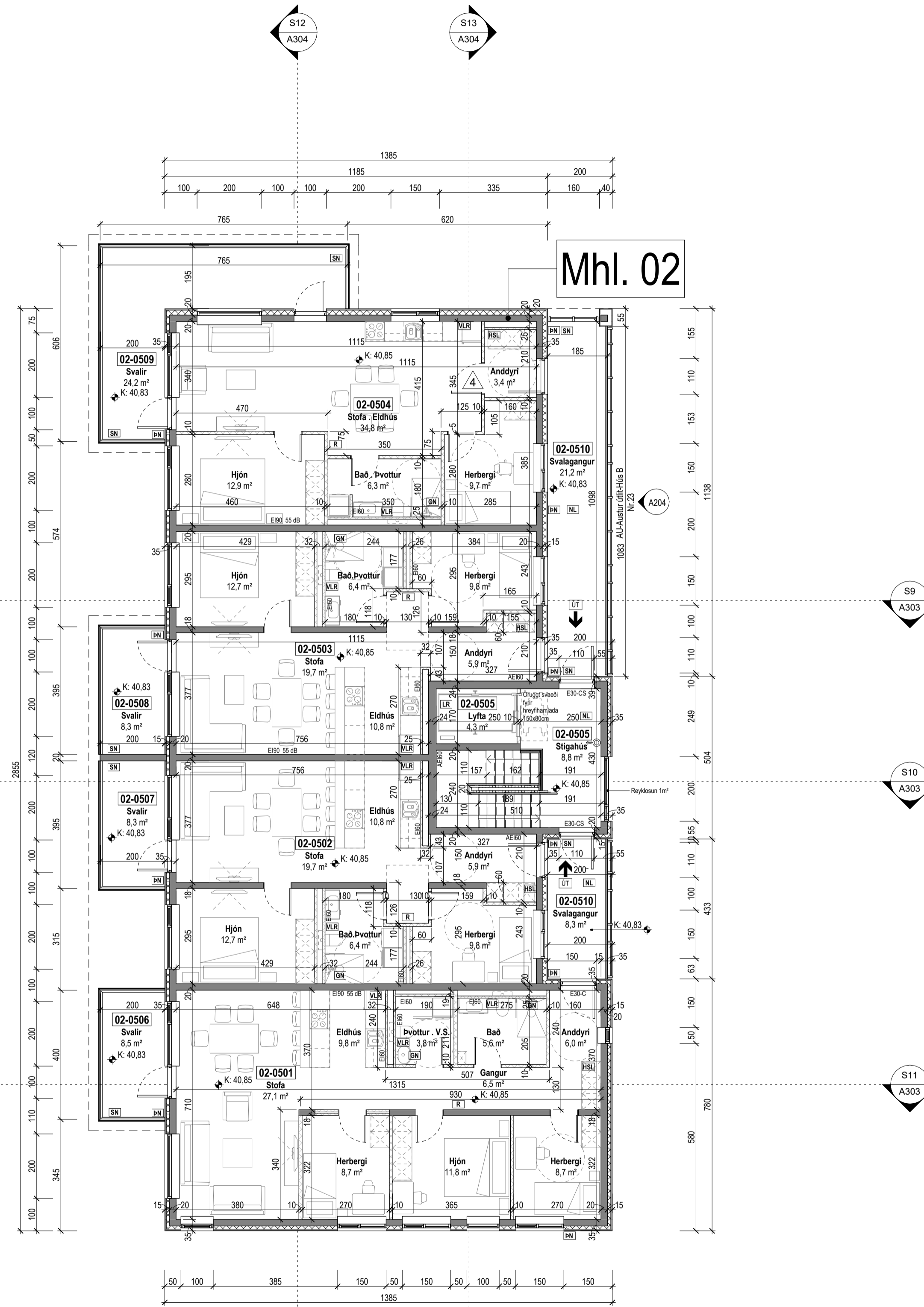
Grunnmynd 5.hæð 1: 100
