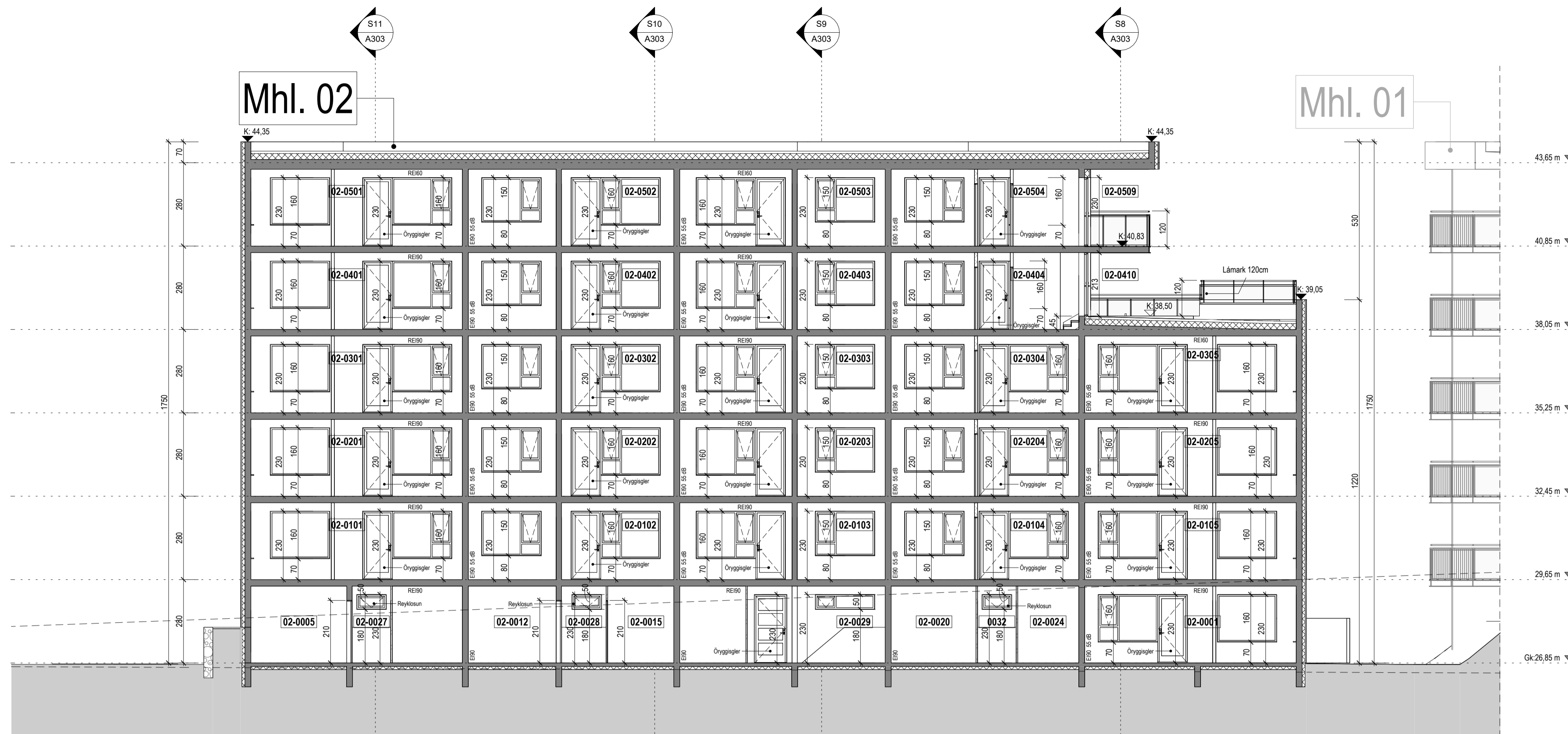
Snið 12 1:100
