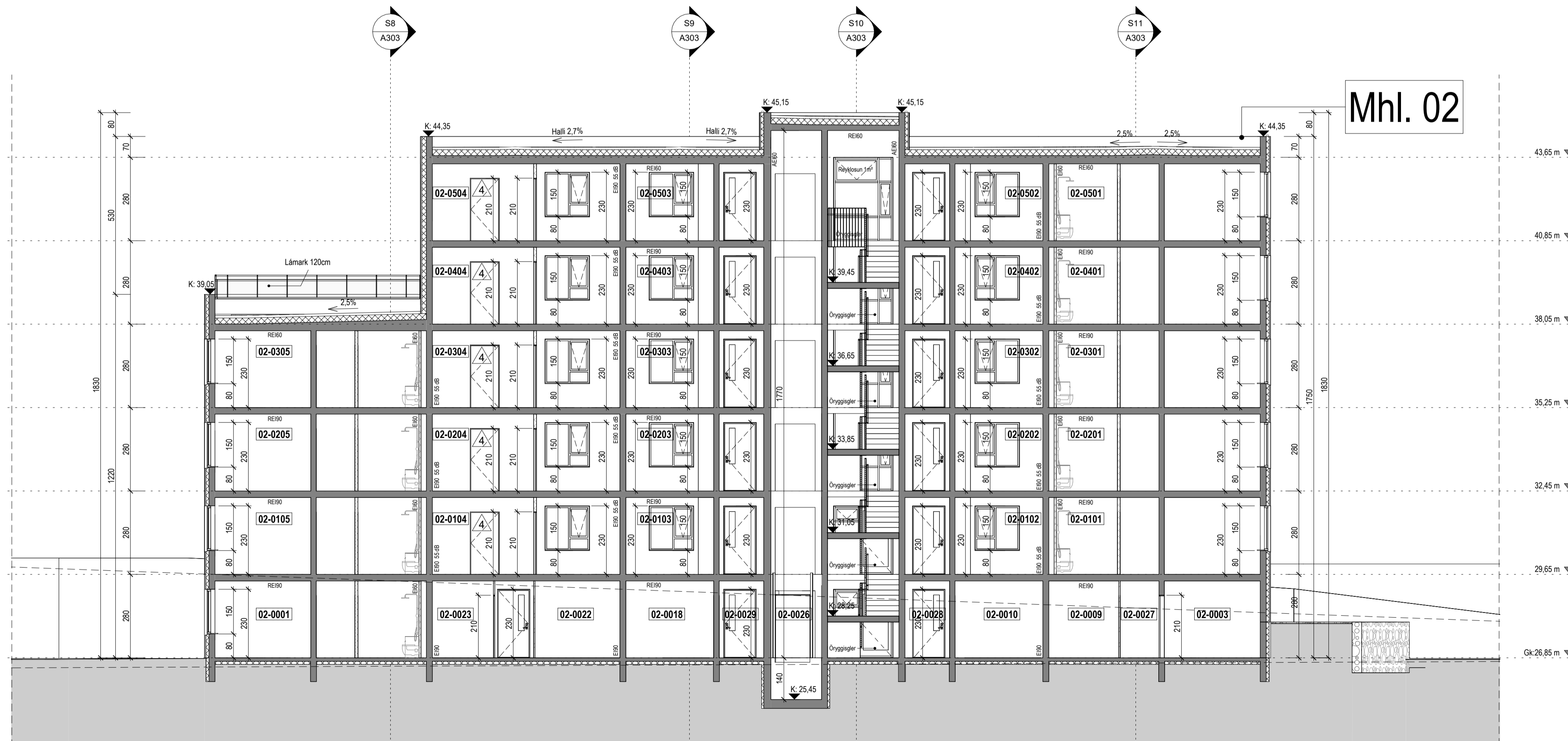
Snið 13 1:100
